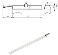
Technische Daten Philips LED Tragschiene Coreline LL212X 49W 8000lm 37x71D - 840 | 1130mm - 5-polig
